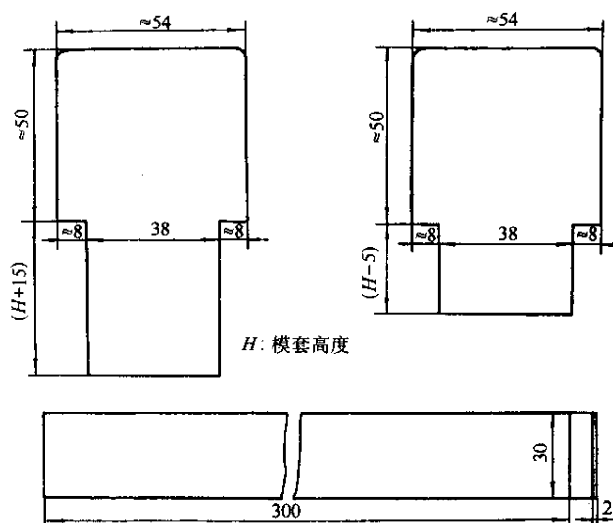
图 3 典型的播料器和金属刮平直尺
