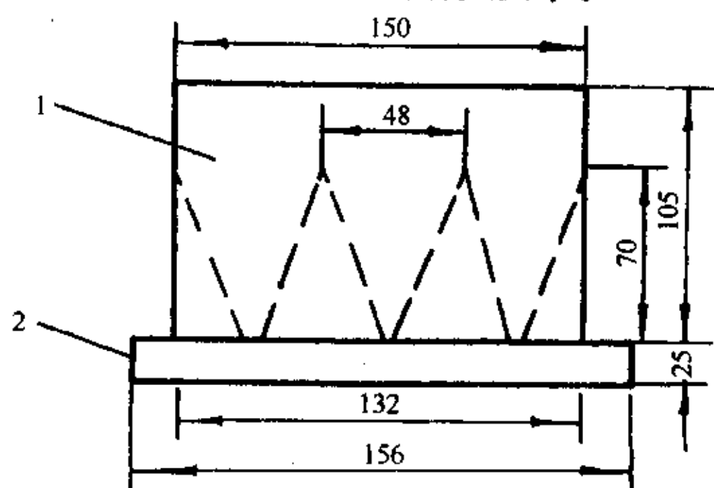
图8 下料漏斗
