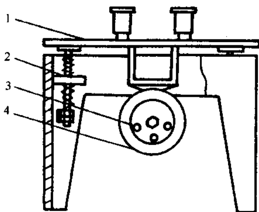
图7 胶砂振动台
