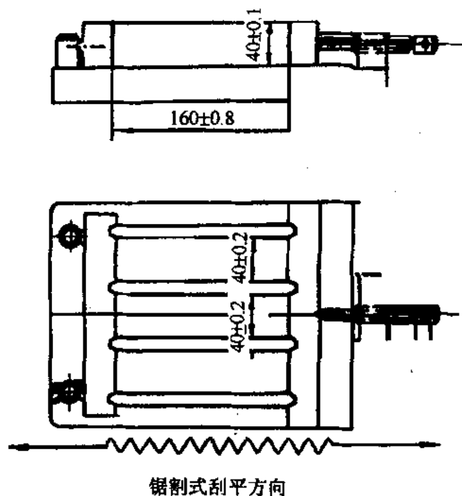
图 2 典型的试模
