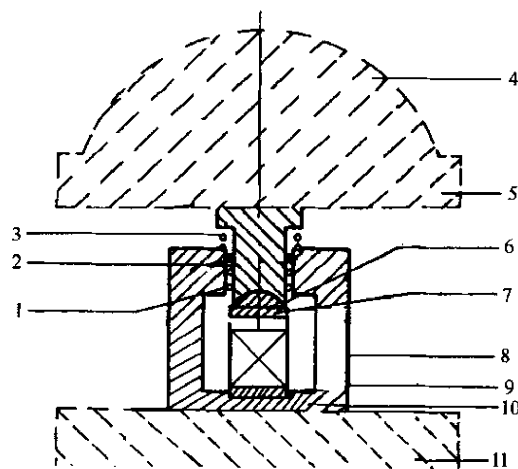
图 6 典型的抗压强度试验夹具
